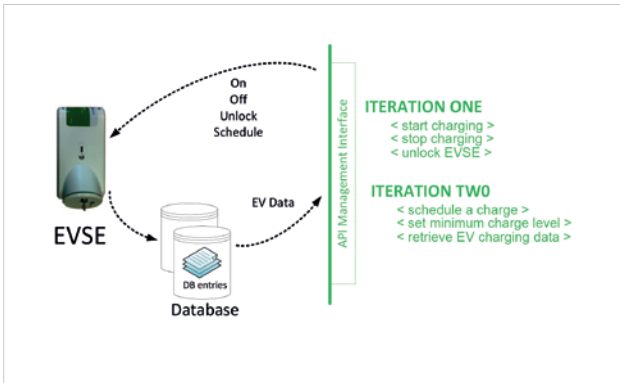
Figure 26: FINESCE EVSE API
